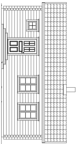
FASAD B 1:100 (A3)
