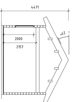
SEKTION A-A (PLATTÅ PÅ MARK) 1:100 (A3)
