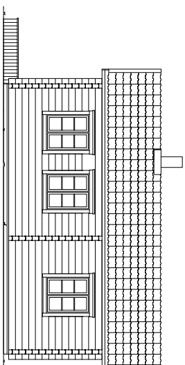
FASAD D 1:100 (A3)
