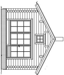
FASAD C 1:100 (A3)
