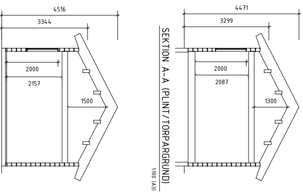
SEKTION A-A (PLATTÅ PÅ MARK) 1:100 (A3)
