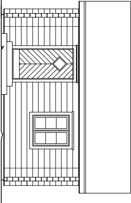
ENTRÉFASAD 2
