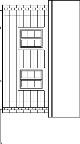
LÅNGFASAD 4
